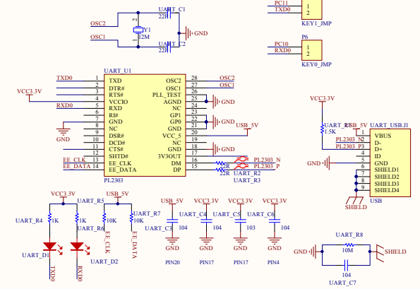
UART0
